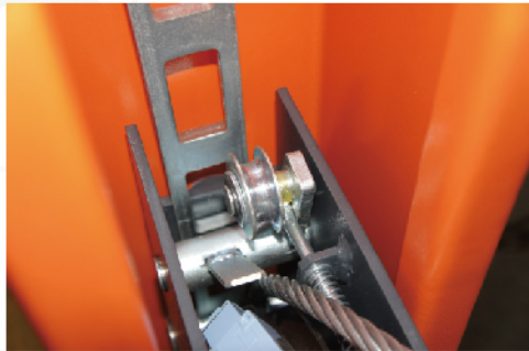
保险锁齿
