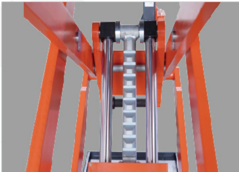
机械保险装置
