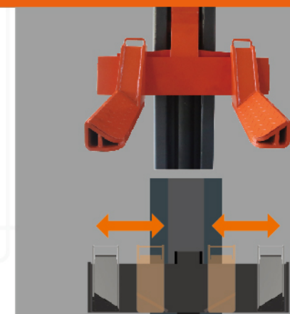
可调节轮架, 适应大多数轮胎尺寸
