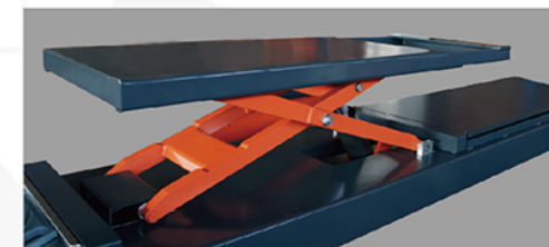
二次举升小车(子剪举升吨位4000kg)
